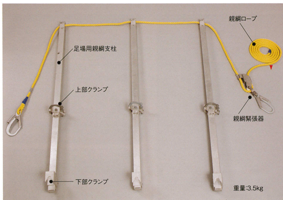
〔形状・寸法図〕
