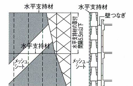
図1 鋼管足場への設置例
